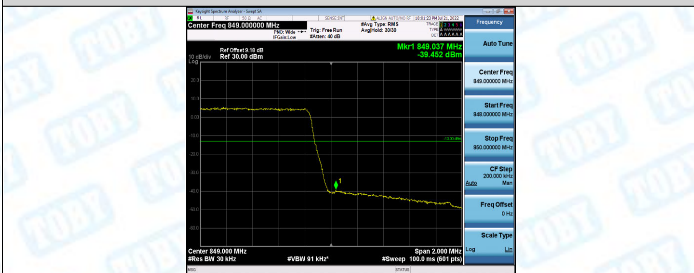
Band5-3MHz-QPSK-20415-1RB#0
