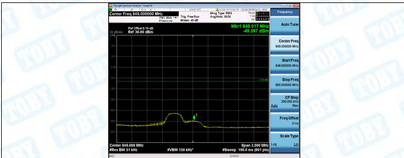
Band5-3MHz-QPSK-20635-1RB#14
