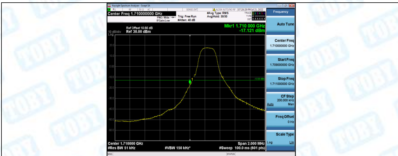
Band4-3MHz-QPSK-19965-1RB#14
