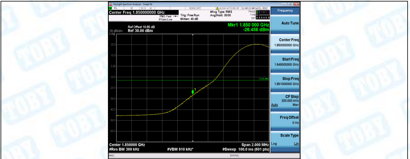
Band2-15MHz-16QAM-18675-1RB#74
