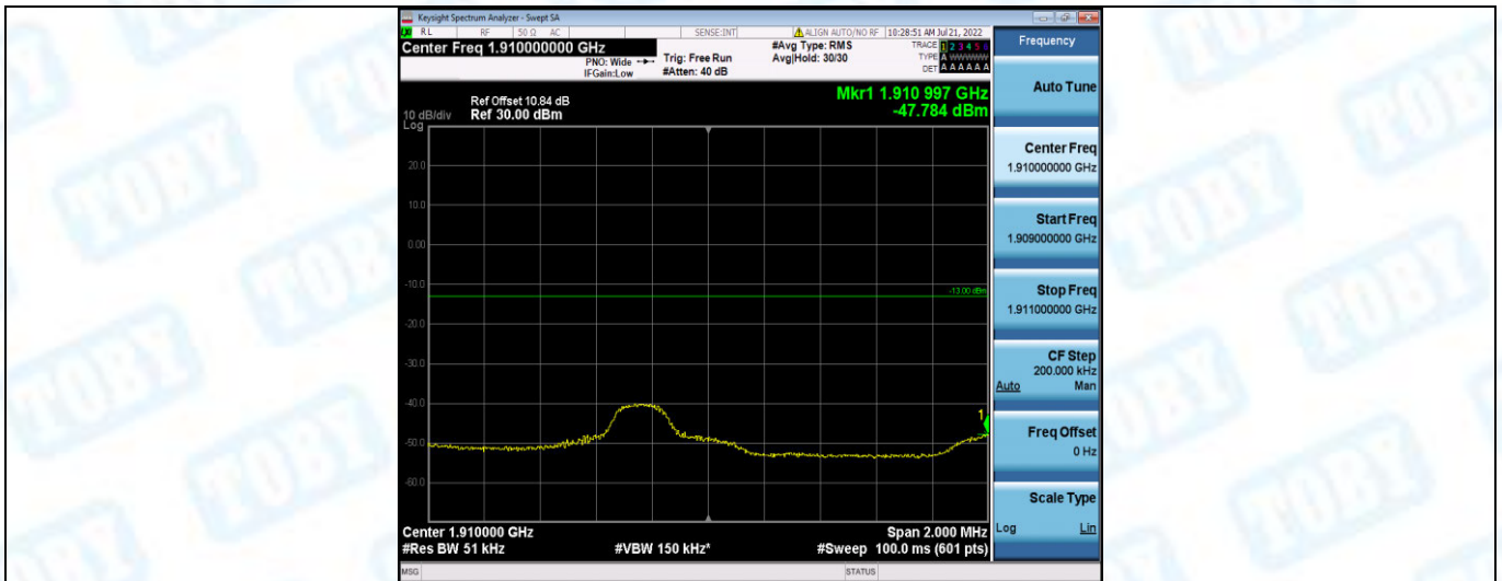
Band2-3MHz-QPSK-19185-1RB#14
