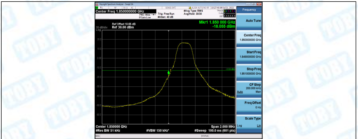
Band2-3MHz-QPSK-18615-1RB#14
