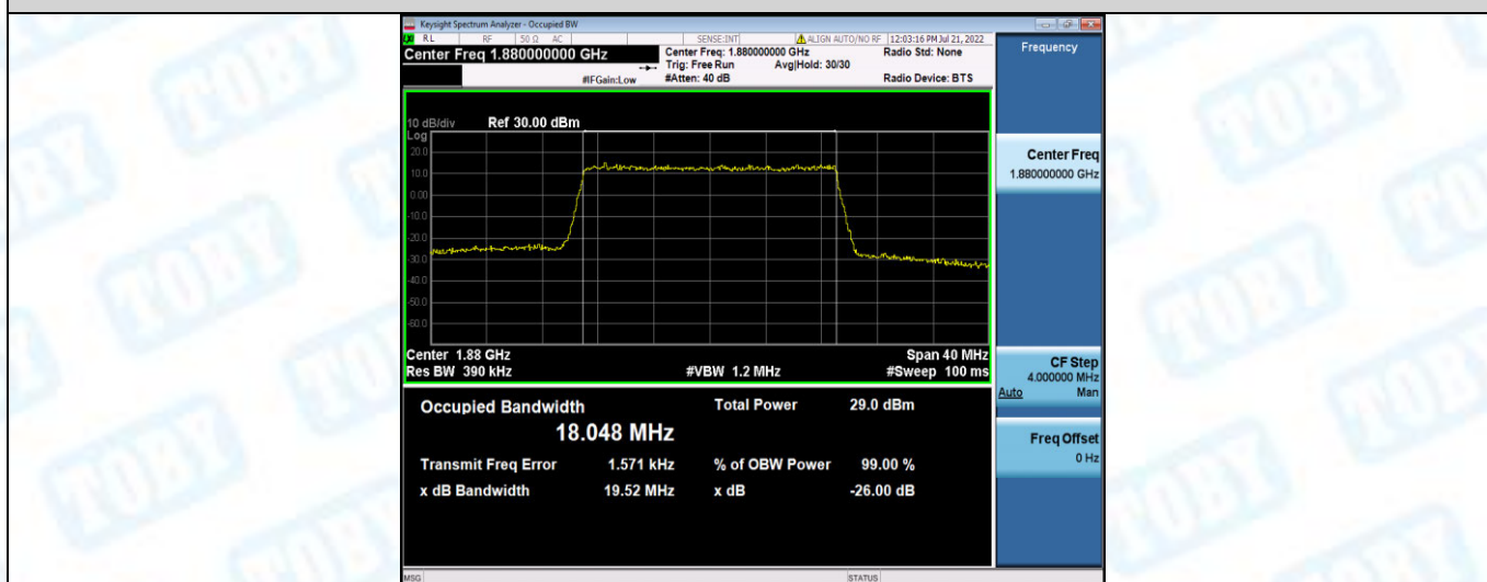
Band2-20MHz-16QAM-19100-100RB#0
