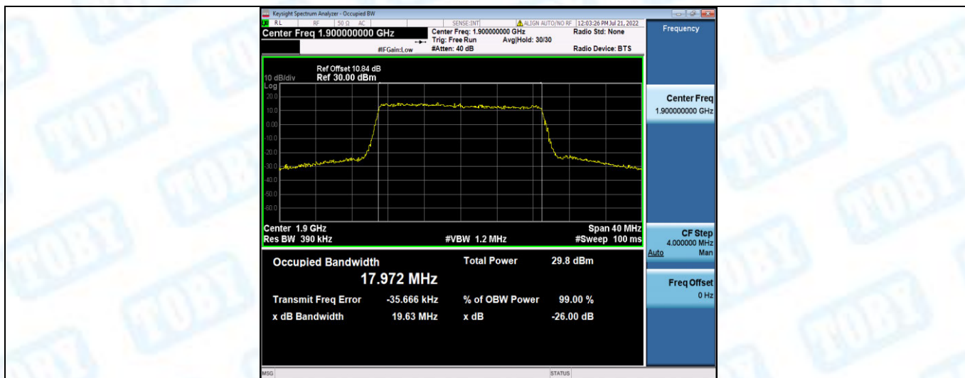
Band2-20MHz-16QAM-18700-100RB#0
