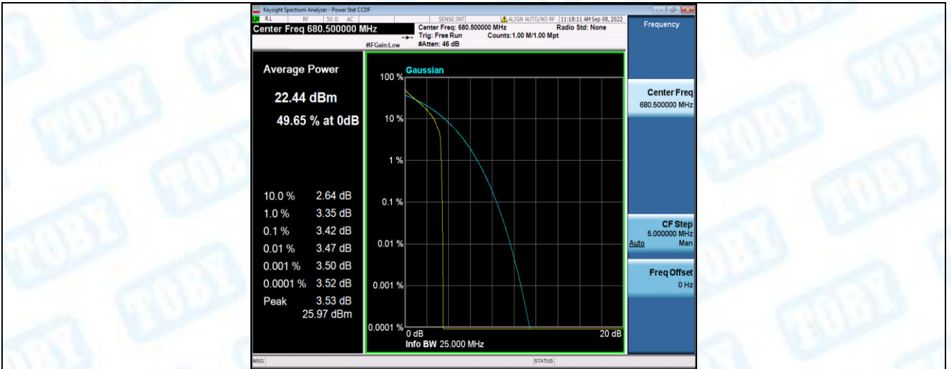
Band71-5MHz-QPSK-133297-25RB#0
