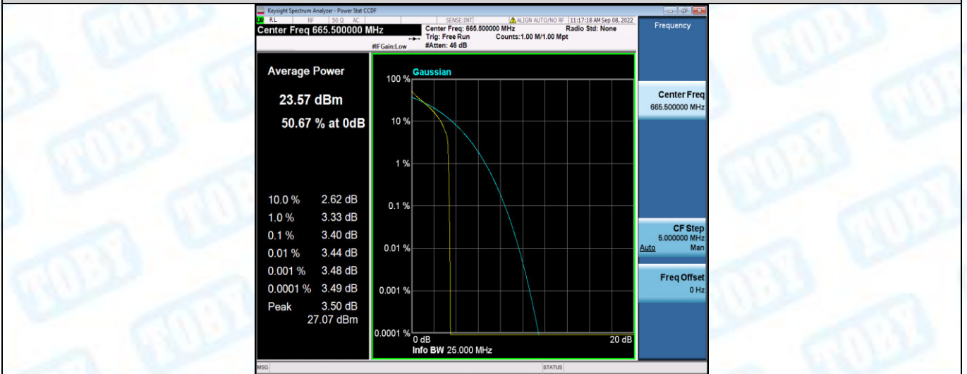
Band71-5MHz-QPSK-133147-25RB#0
