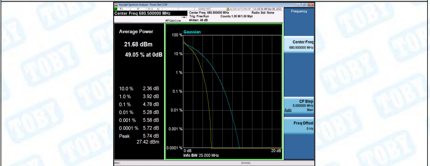
Band71-5MHz-QPSK-133447-1RB#0
