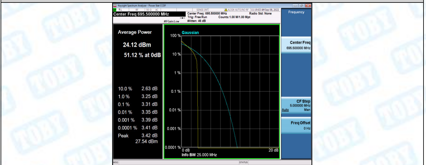
Band71-5MHz-QPSK-133447-25RB#0
