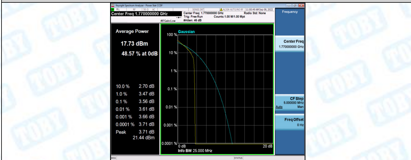
Band66-20MHz-QPSK-132572-100RB#0
