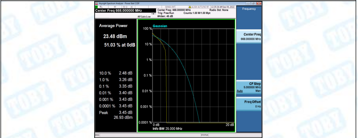
Band71-10MHz-QPSK-133172-50RB#0
