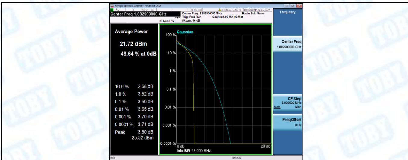
Band25-3MHz-QPSK-26365-15RB#0
