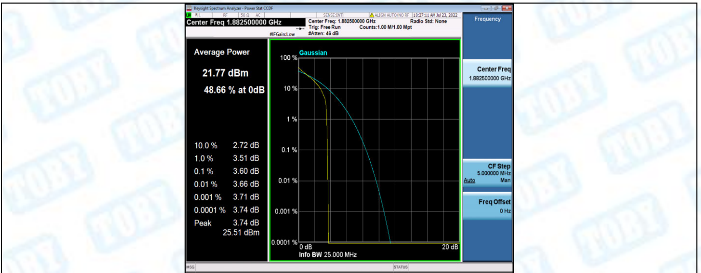
Band25-5MHz-QPSK-26365-25RB#0
