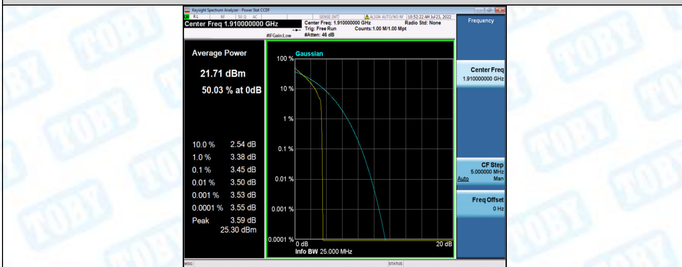
Band25-10MHz-QPSK-26640-50RB#0
