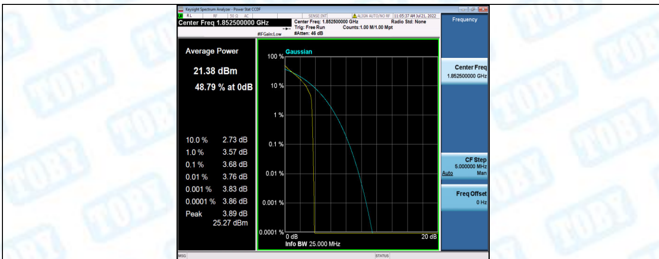
Band2-5MHz-QPSK-18625-25RB#0
