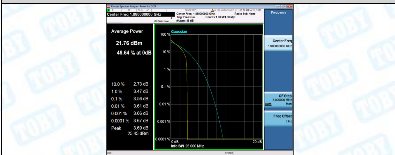
Band2-5MHz-QPSK-18900-25RB#0
