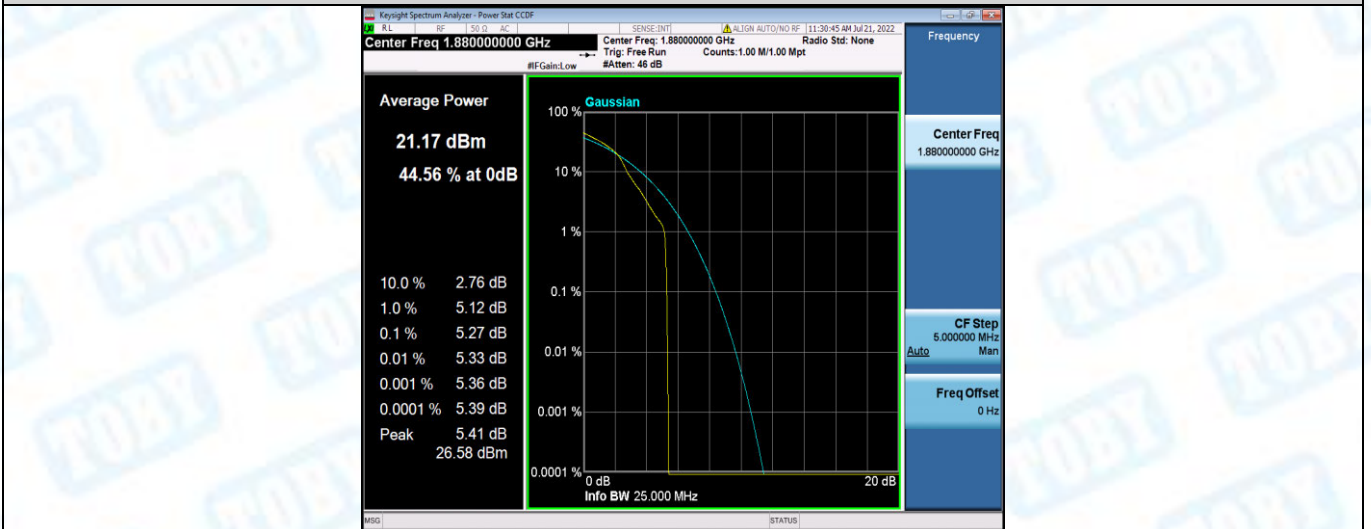
Band2-10MHz-16QAM-18900-50RB#0
