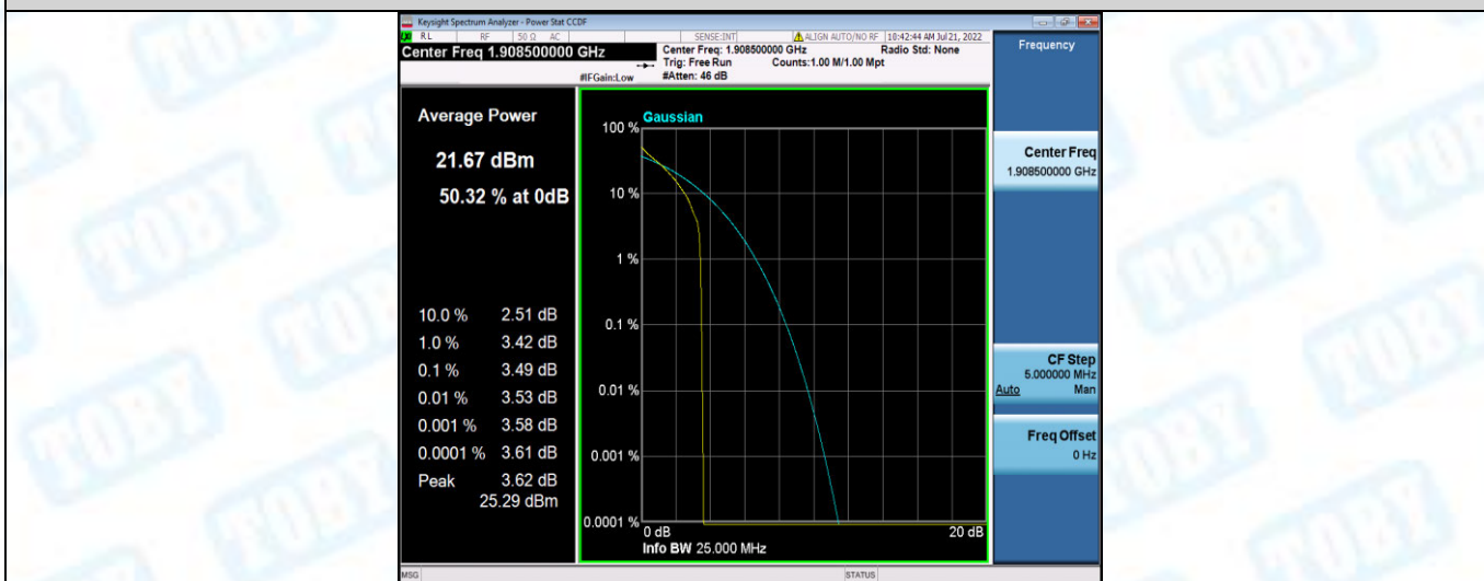
Band2-3MHz-QPSK-19185-15RB#0
