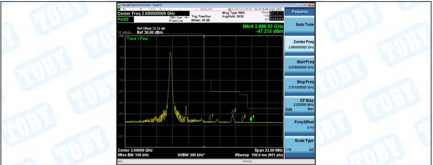
Band41-5MHz-16QAM-41565-1RB#24
