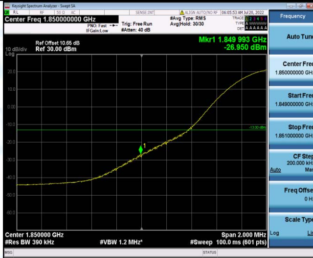
Band25-20MHz-QPSK-26140-1RB#99
