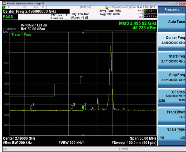
Band41-10MHz-QPSK-39700-50RB#0
