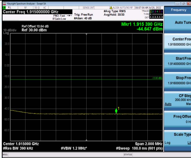
Band25-20MHz-QPSK-26590-1RB#99
