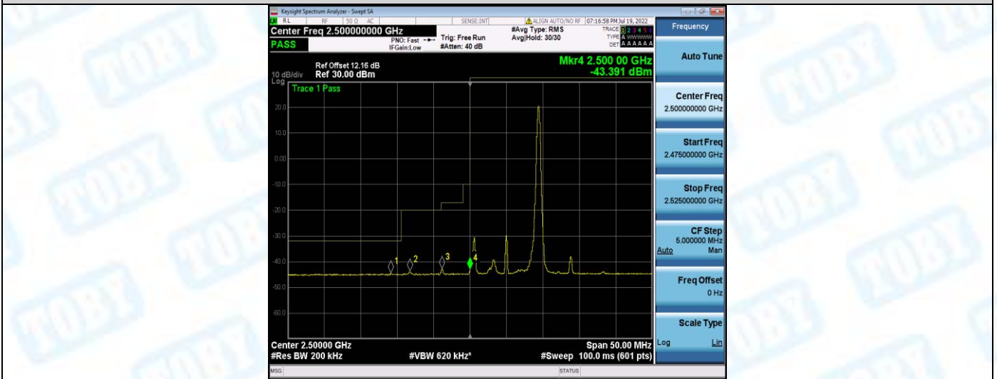
Band7-10MHz-QPSK-20800-50RB#0
