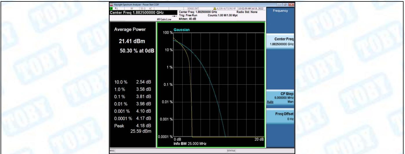
Band25-1.4MHz-QPSK-26365-6RB#0
