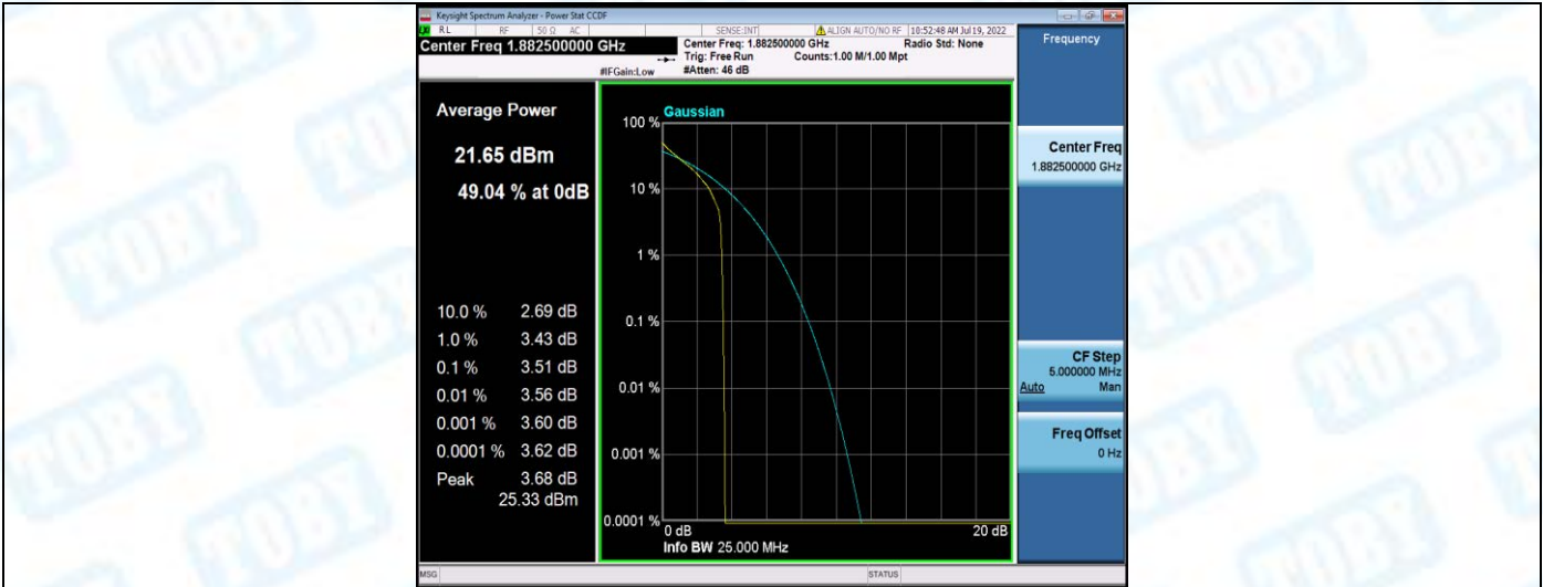
Band25-5MHz-QPSK-26365-25RB#0
