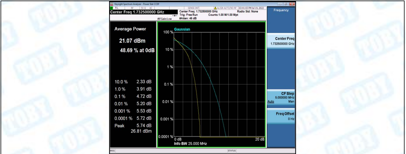
Band4-10MHz-QPSK-20350-1RB#0
