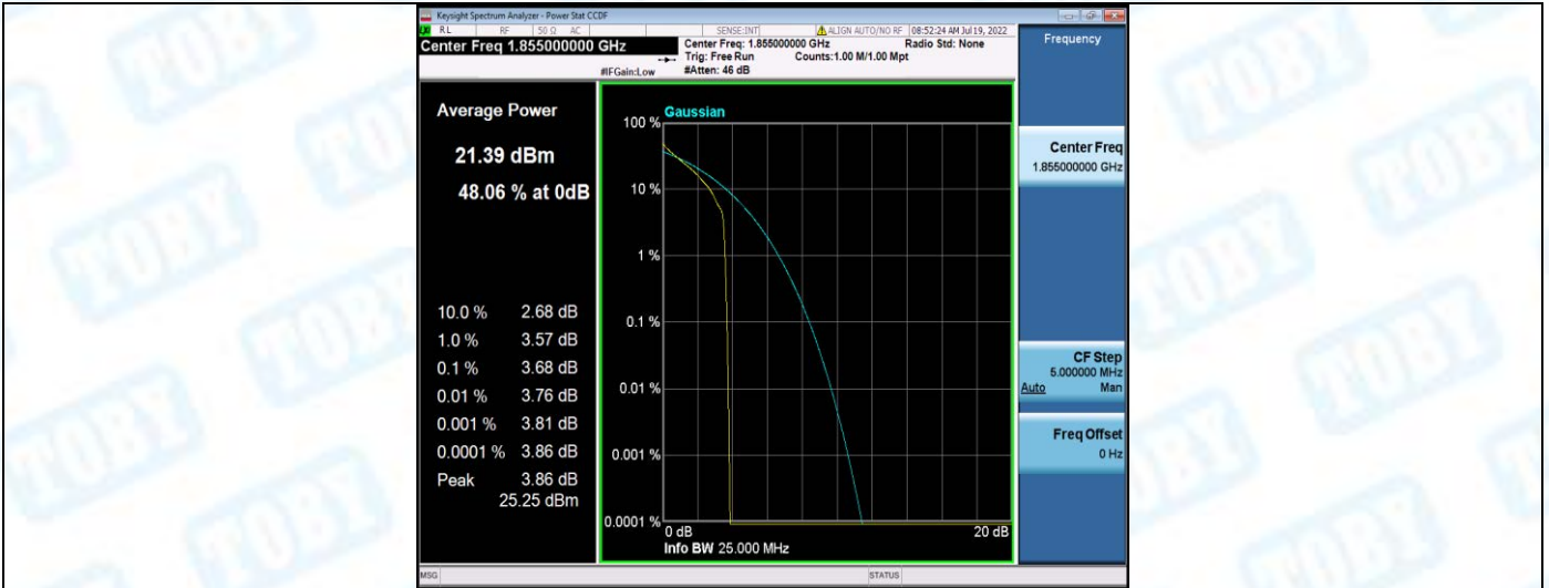
Band2-10MHz-QPSK-18650-50RB#0
