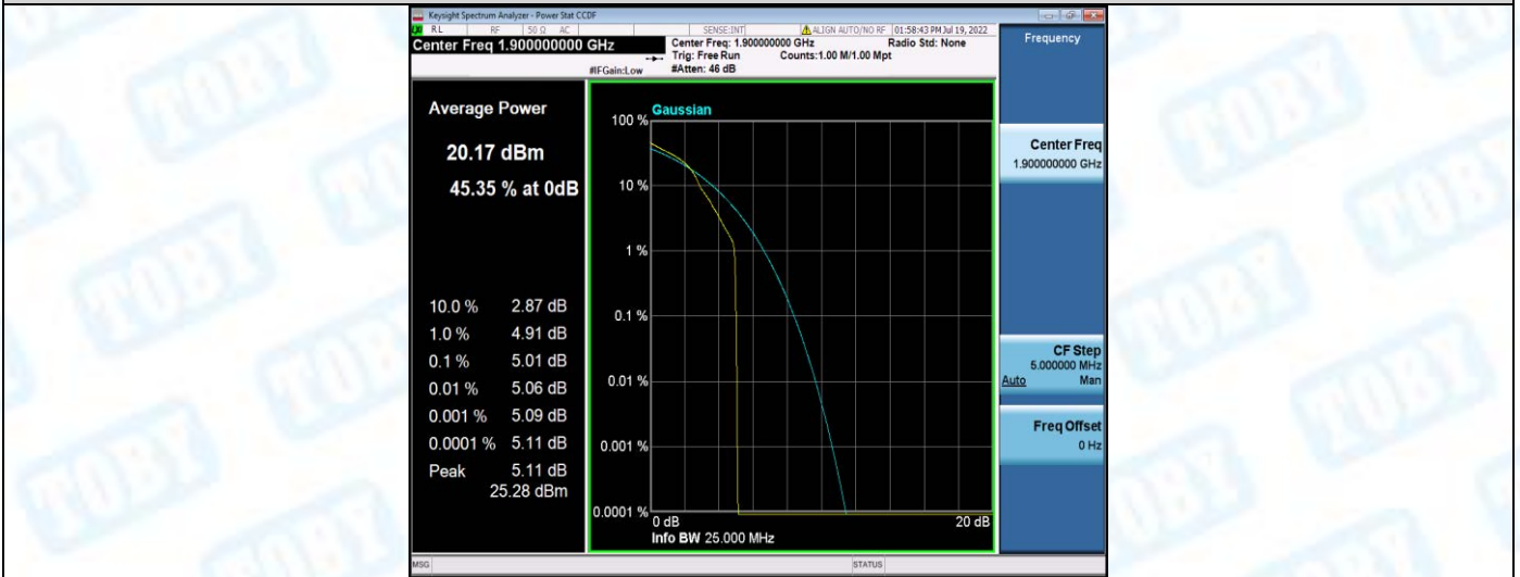
Band2-20MHz-16QAM-19100-100RB#0
