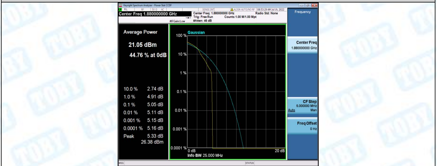
Band2-10MHz-16QAM-18900-50RB#0
