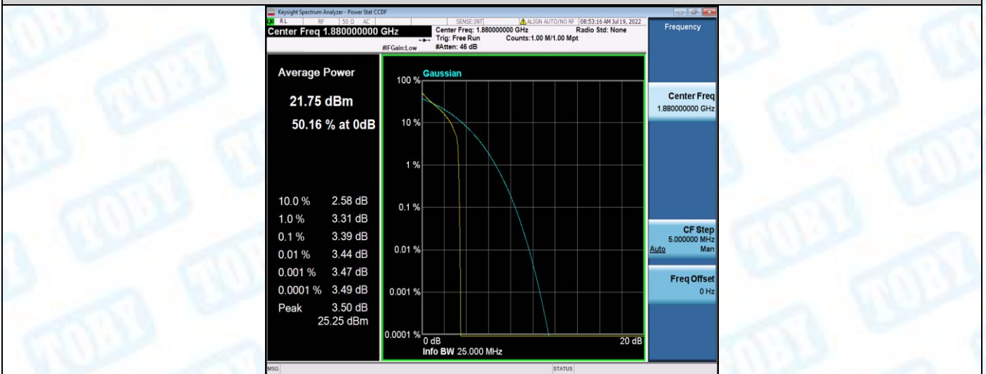
Band2-10MHz-QPSK-18900-50RB#0
