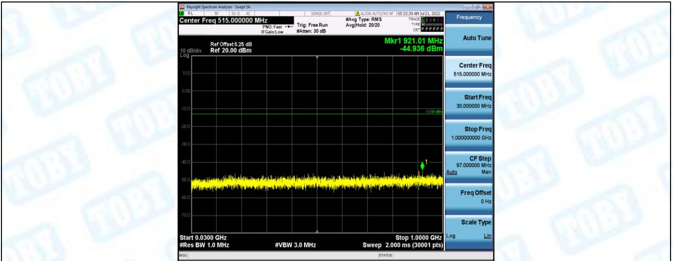
Band4-1312-2-30~1000MHz
