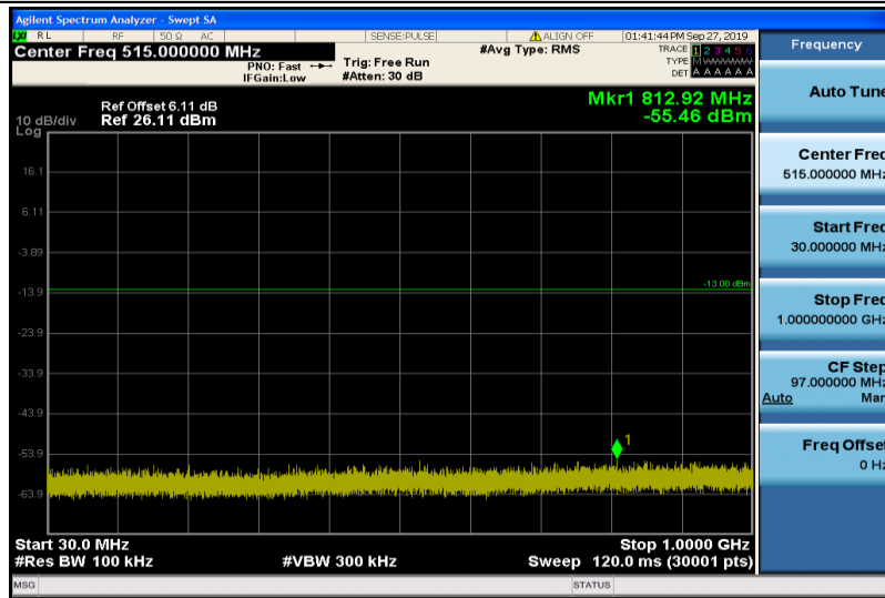
Band2-3MHz-QPSK-18900-1RB#0-30~1000MHz
