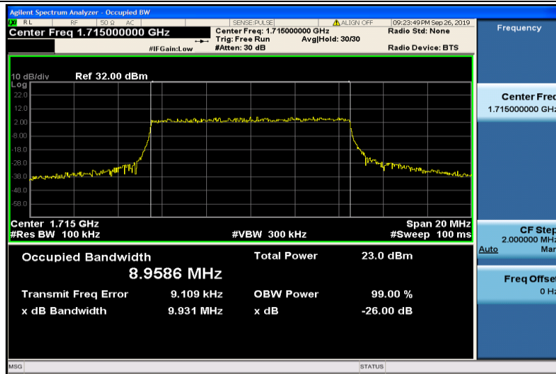
Band4-10MHz-QPSK-20000-50RB#0-8.9586
