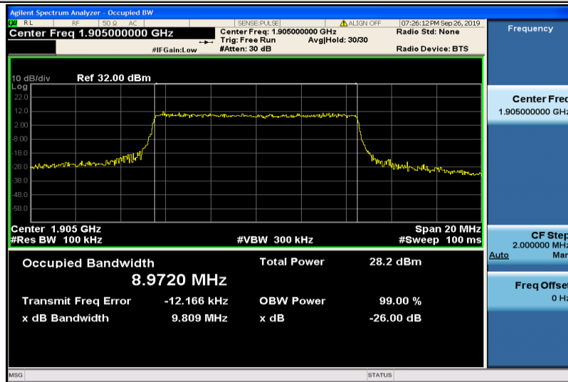
Band2-10MHz-QPSK-19150-50RB#0-8.9720
