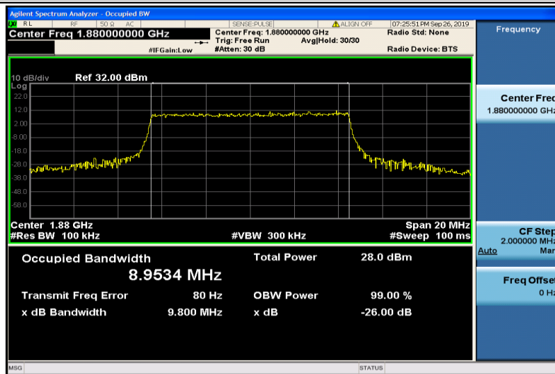
Band2-10MHz-QPSK-18900-50RB#0-8.9534
