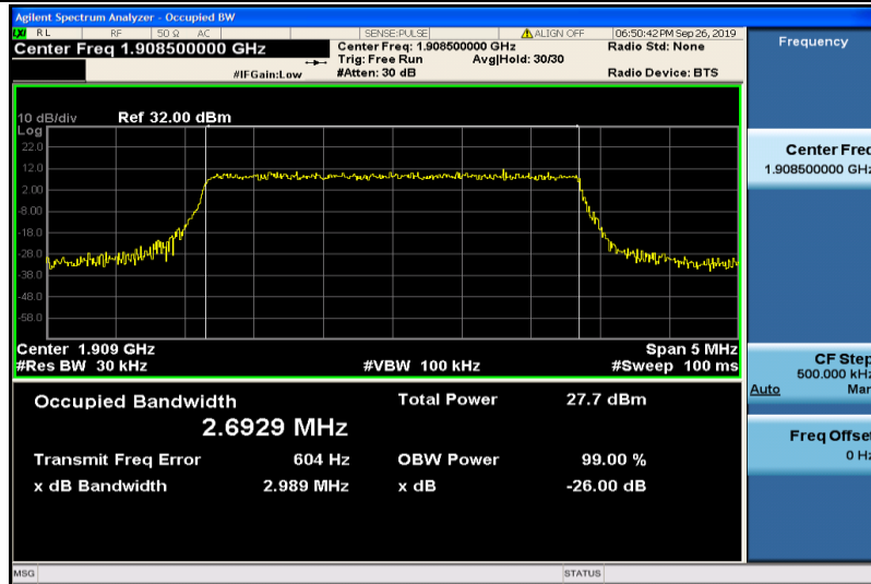
Band2-3MHz-QPSK-19185-15RB#0-2.6929
