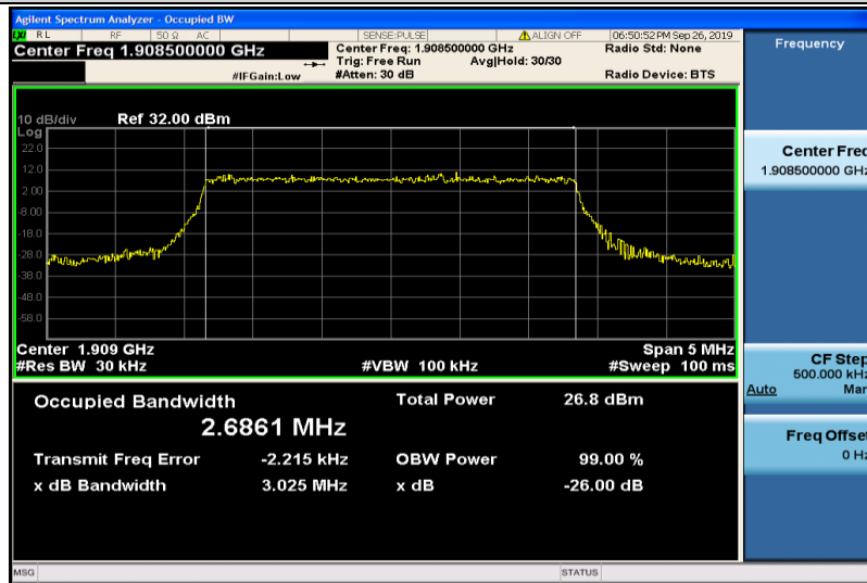
Band2-3MHz-16QAM-19185-15RB#0-2.6861
