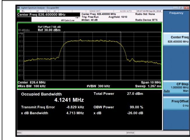
WCDMA 850-LCH
