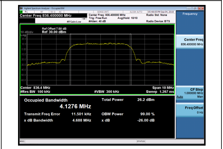
WCDMA 850-MCH
