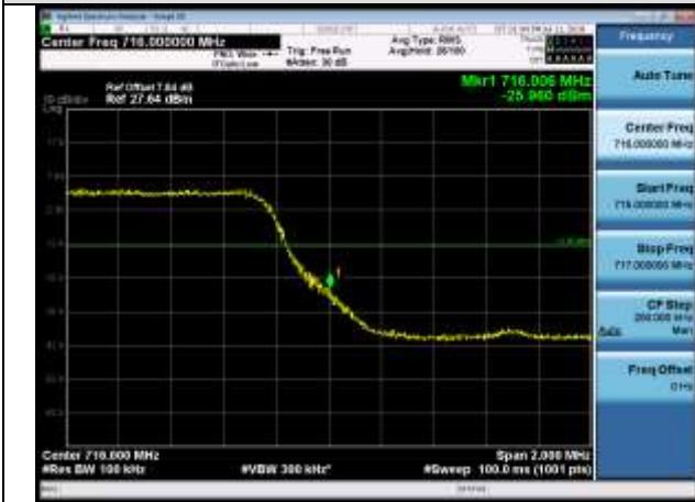
HCH_QPSK_25RB#0
