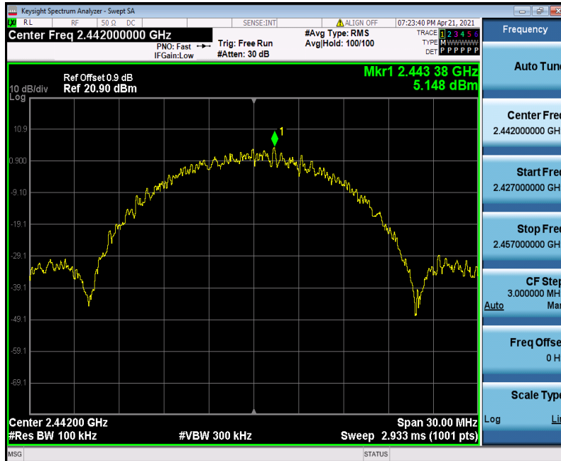
11B_Ant1_2442_0~Reference
