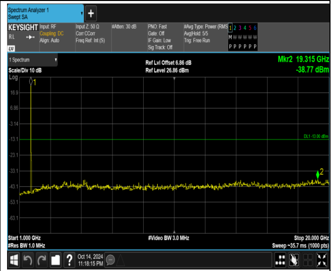
Band66-20MHz-QPSK-132322-1RB#0-Range2:1000~20000MHz
