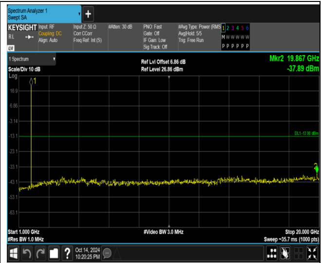
Band66-20MHz-QPSK-132072-1RB#0-Range2:1000~20000MHz
