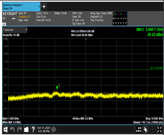
Band26-1.4MHz-QPSK-26797-1RB#0-Range2:1000~10000MHz
