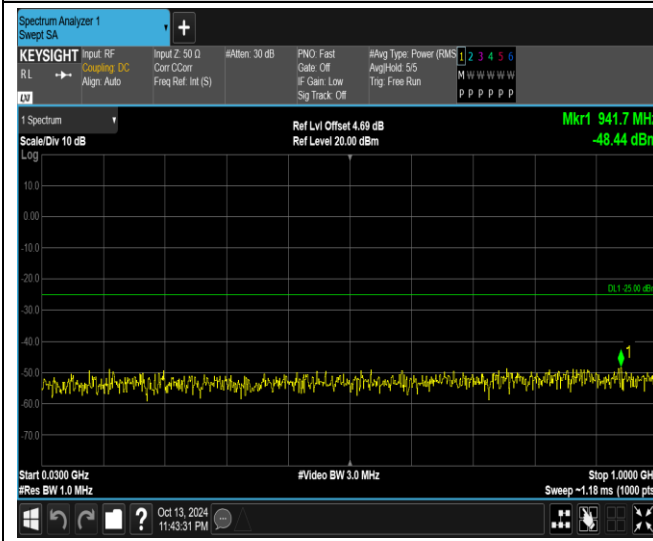
Band7-20MHz-QPSK-21350-1RB#0-Range1:30~100 0MHz
