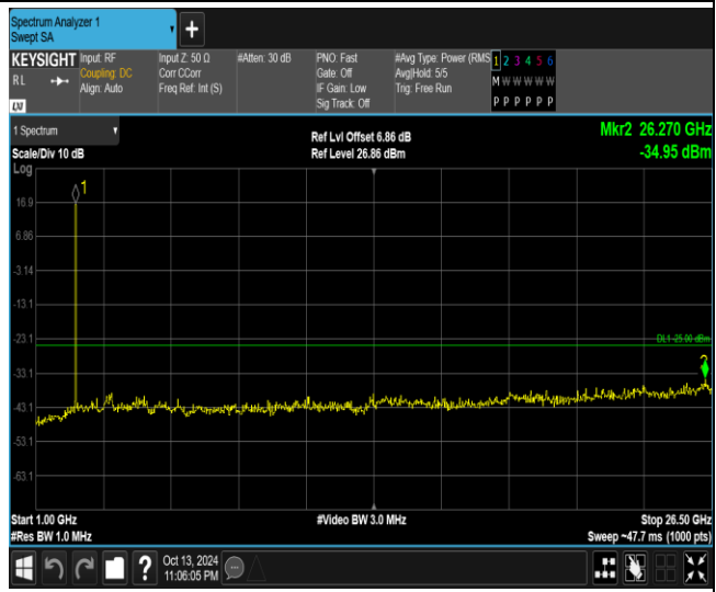
Band7-5MHz-QPSK-21100-1RB#0-Range2:1000~26 500MHz
