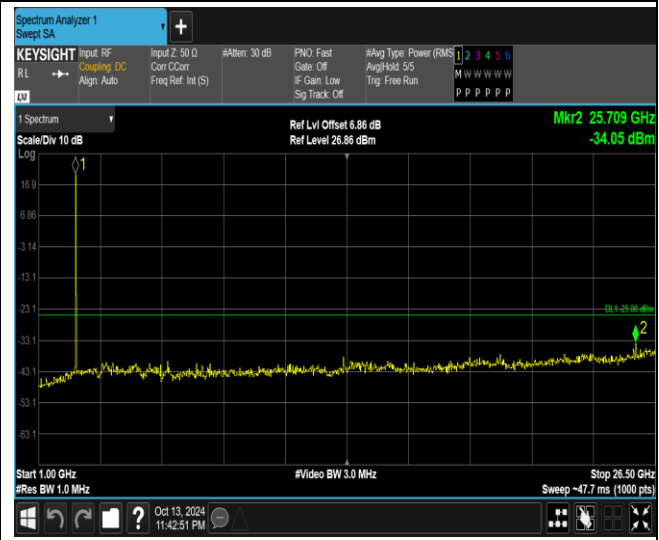
Band7-20MHz-QPSK-21350-1RB#0-Range2:1000~2 6500MHz
