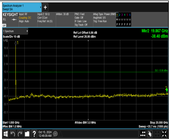
Band2-20MHz-16QAM-18900-1RB#0-Range2:1000~20000MHz
