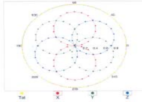
f=1800 MHz,R22
