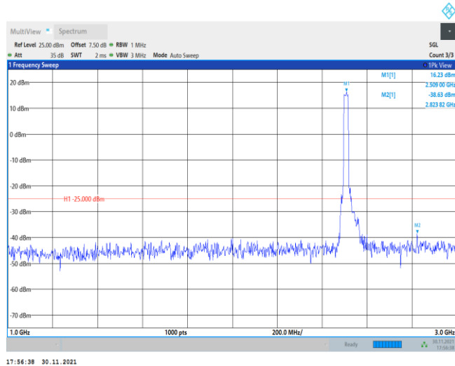
Band41-20MHz-QPSK-39750-1RB#0-Range2:1000~3000MHz
