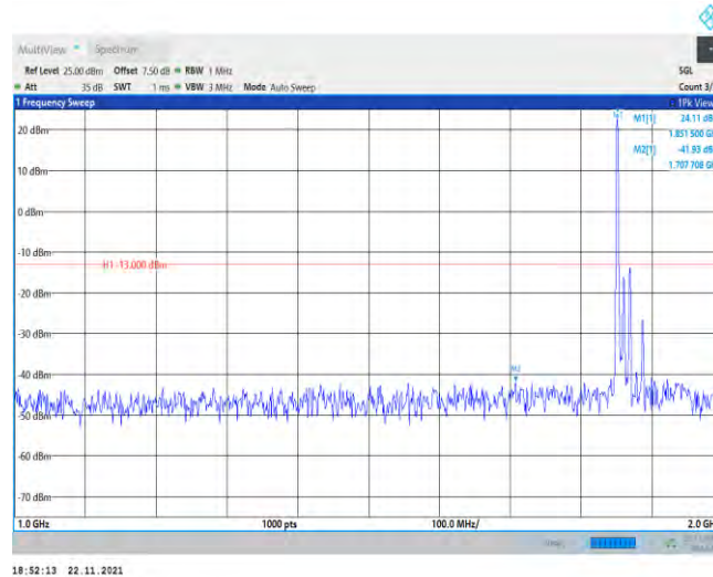
Band25-20MHz-QPSK-26140-1RB#0-Range2:1000~2000MHz
