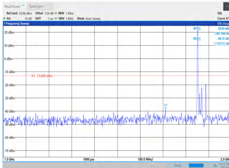
Band2-20MHz-QPSK-18700-1RB#0-Range2:1000~2000MHz
