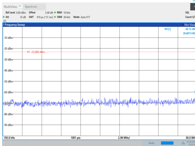
Band71-20MHz-QPSK-133222-1RB#0-Range2:0.15~30MHz
