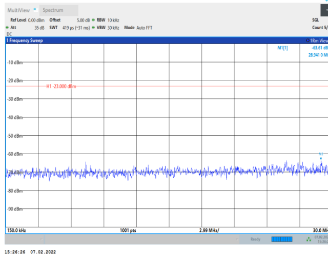
Band26-10MHz-QPSK-26740-1RB#0-Range2:0.15~30MHz
