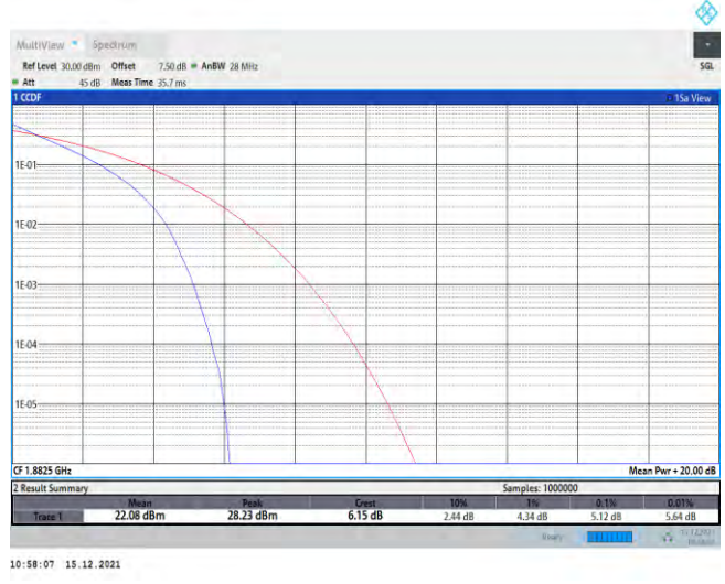
Band25-20MHz-QPSK-26365-100RB#0
