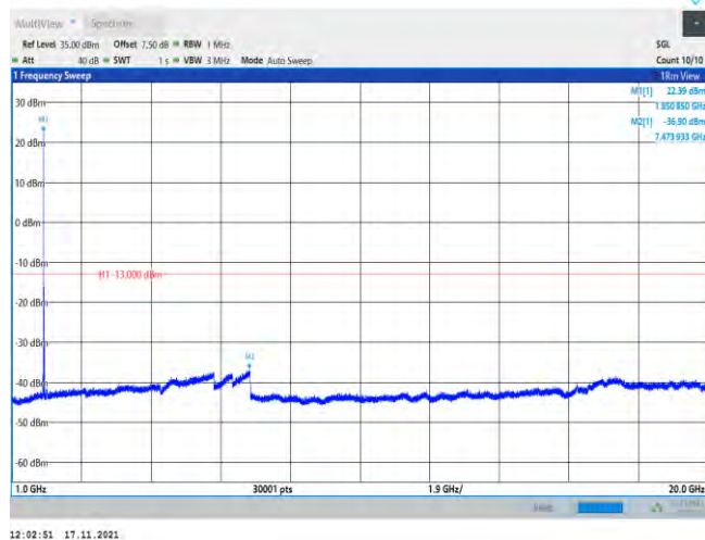
Band2-20MHz-QPSK-18700-1RB#0-Range2:1000~20000MHz
