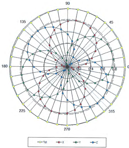
f=600 MHz, TEM
