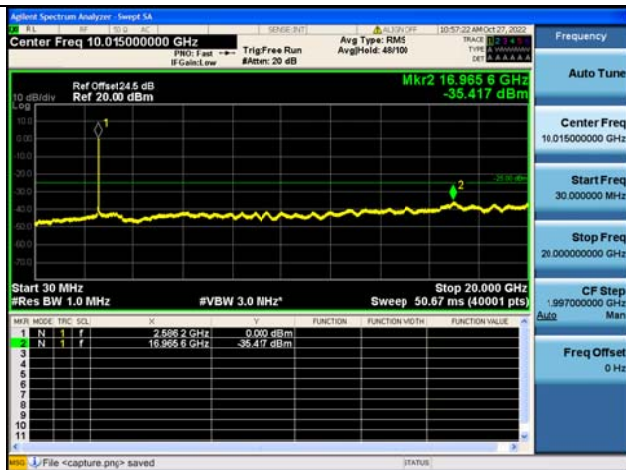
Band41C-30M-20G / 20MHz+15MHz /100RB+75RB/ QPSK / Mid CH
