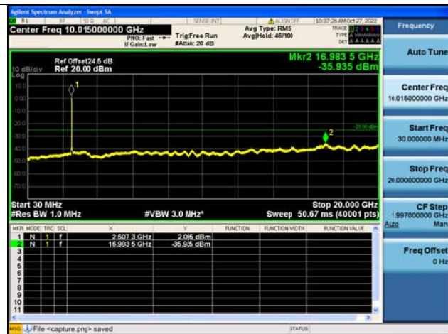
Band41C-30M-20G / 20MHz+20MHz / 100RB+100RB/ QPSK / LOW CH
