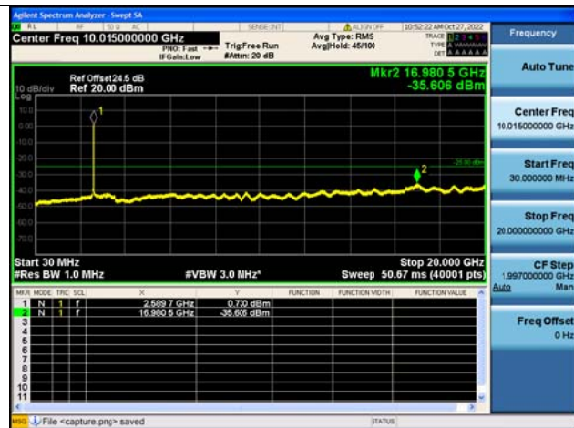
Band41C-30M-20G / 20MHz+10MHz /100RB+50RB/ QPSK / Mid CH
