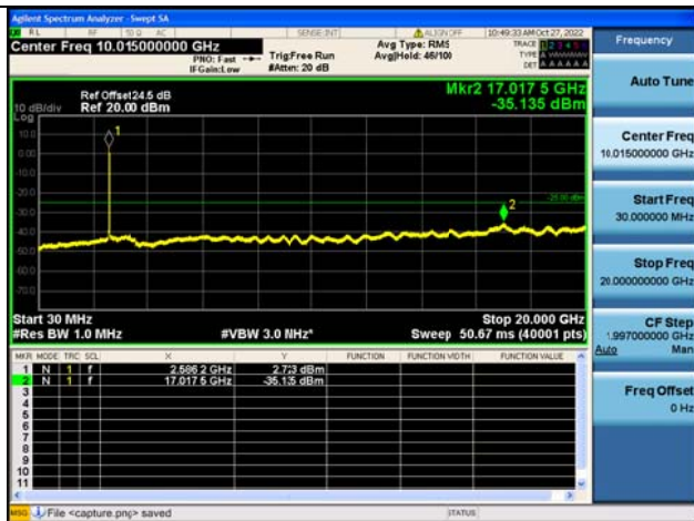
Band41C-30M-20G / 10MHz+20MHz /50RB+100RB/ QPSK / Mid CH
