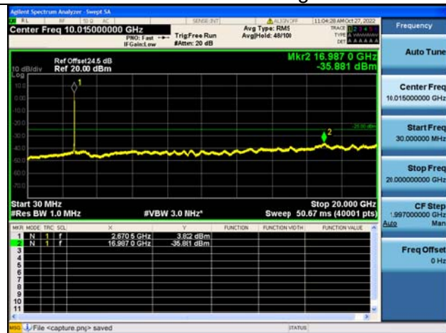
Band41C-30M-20G / 10MHz+15MHz /50RB+75RB/ QPSK / High CH
