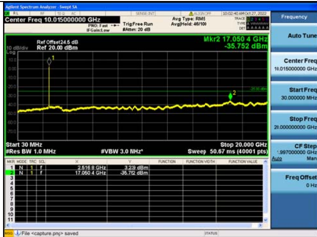
Band41C-30M-20G / 20MHz+5MHz / 100RB+25RB / QPSK / LOW CH
