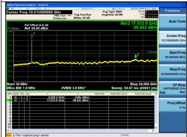
Band7C-30M-20G / 20MHz+15MHz / 100RB+75RB / QPSK / Mid CH
