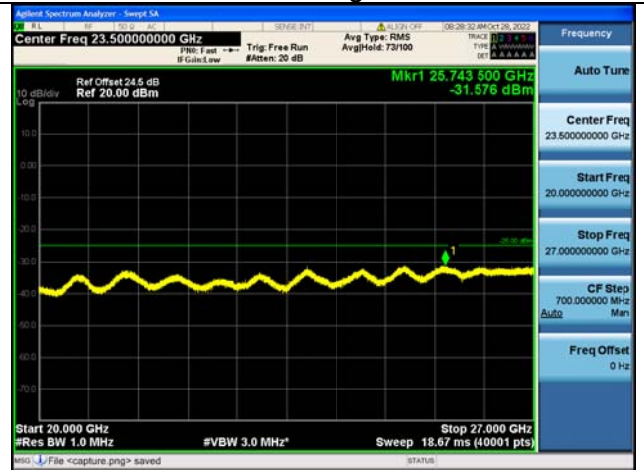
Band7C-20G-27G / 20MHz+15MHz / 100RB+75RB / QPSK / High CH
