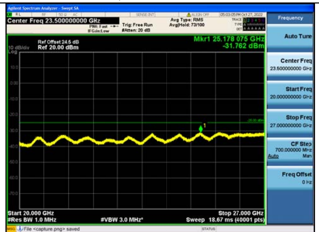
Band7C-20G-27G / 20MHz+15MHz / 1RB+1RB / QPSK / Mid CH
