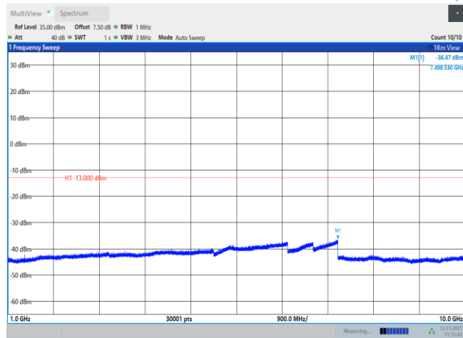
Band71-20MHz-QPSK-133222-1RB#0-Range2:1000~10000MHz
