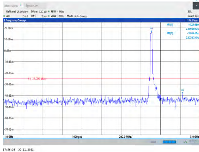
Band41-20MHz-QPSK-39750-1RB#0-Range2:1000~3000MHz
