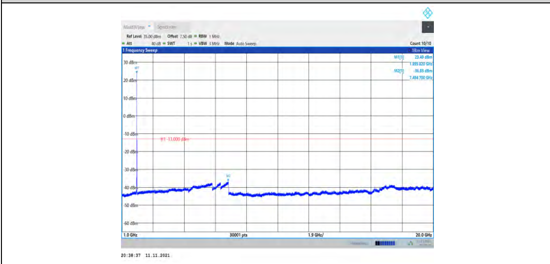
Band25-20MHz-QPSK-26590-1RB#0-Range2:1000~20000MHz
