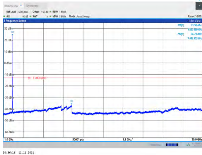
Band25-20MHz-QPSK-26140-1RB#0-Range2:1000~20000MHz
