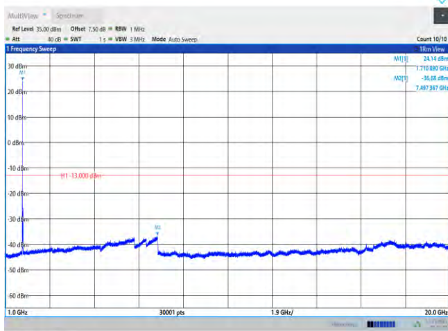
Band4-20MHz-QPSK-20050-1RB#0-Range2:1000~20000MHz
