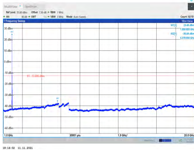
Band2-20MHz-QPSK-18700-1RB#0-Range2:1000~20000MHz
