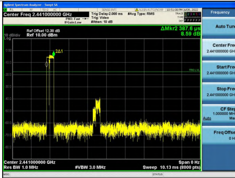
2DH3_Ant1_Hop
