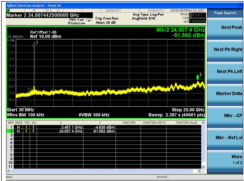
(30MHz to 25GHz, 2457MHz)
