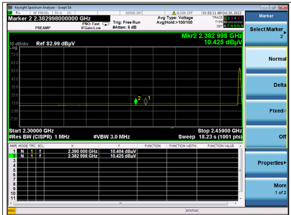
(AVERAGE, 2457MHz)
