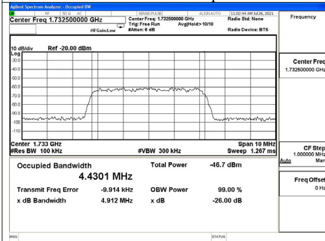
AWS band UL input
