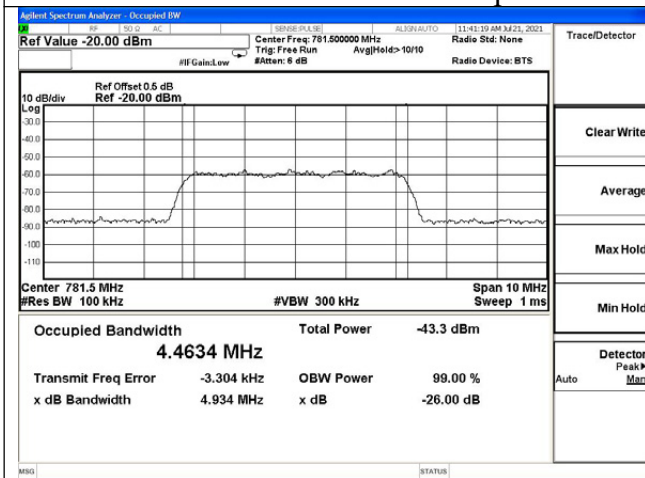
Upper 700MHz band UL input
