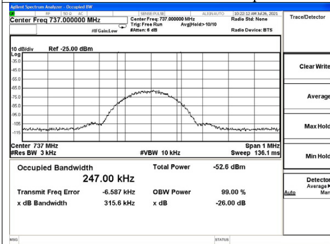
Lower 700MHz band DL input
