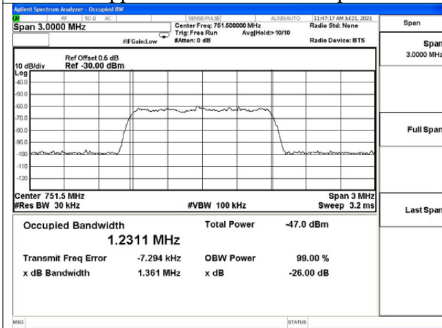
Upper 700MHz band DL input
