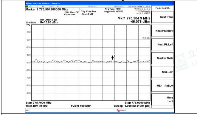
Upper 700MHz band CDMA UL Left Side Pre AGC
