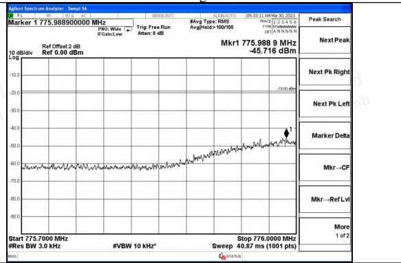
Upper 700MHz band GSM UL Left Side 10dB Above AGC
