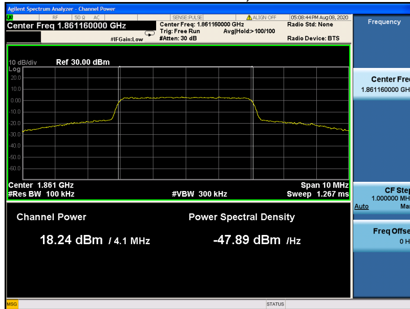
Band2 AWGN, UL
