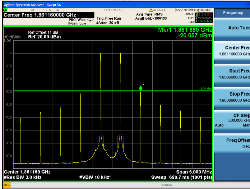
Band2 Pre AGC, UL
