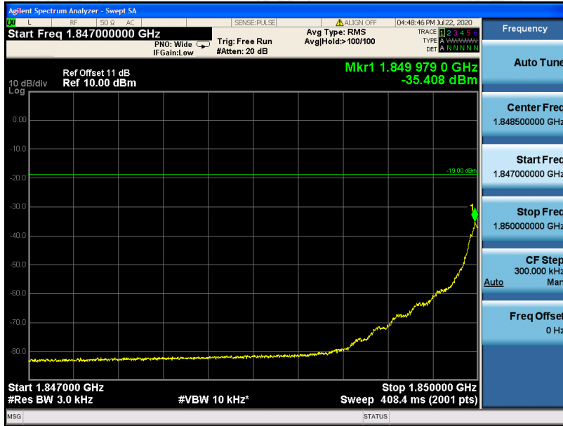
Band2 GSM UL Left Side Max. Input
