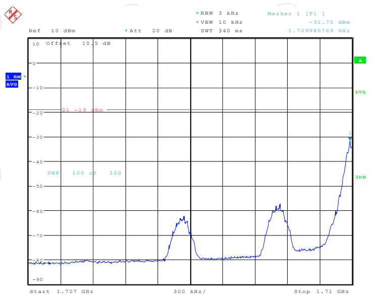
Band4 GSM UL Left Side Max Input
