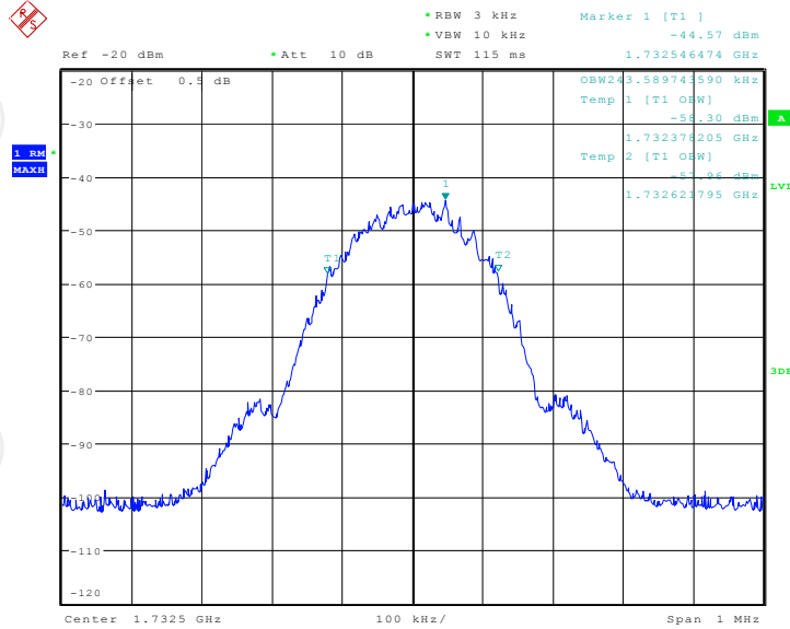
Band4 GSM UL Input
