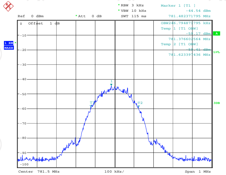
Band13 GSM UL Input
