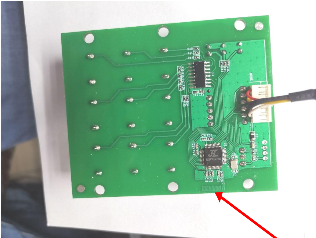
PCB ANT
