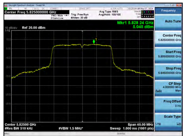
802.11a (CH 165 : 5825 MHz) : Chain 1
