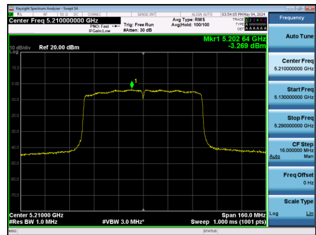
802.11ac VHT80 (CH 42 : 5210 MHz) : Chain 1
