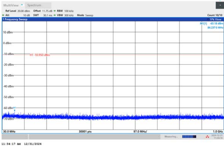
BLE_2M-Ant1-2404-30~1000-PASS
