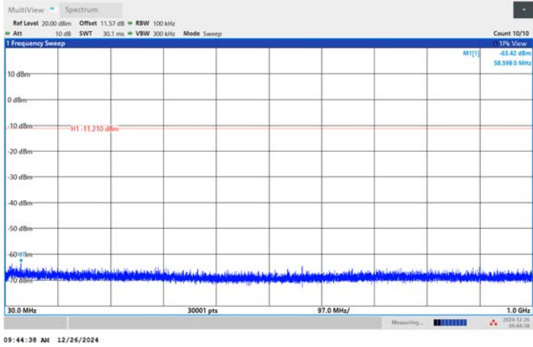
BLE_2M-Ant1-2440-30~1000-PASS
