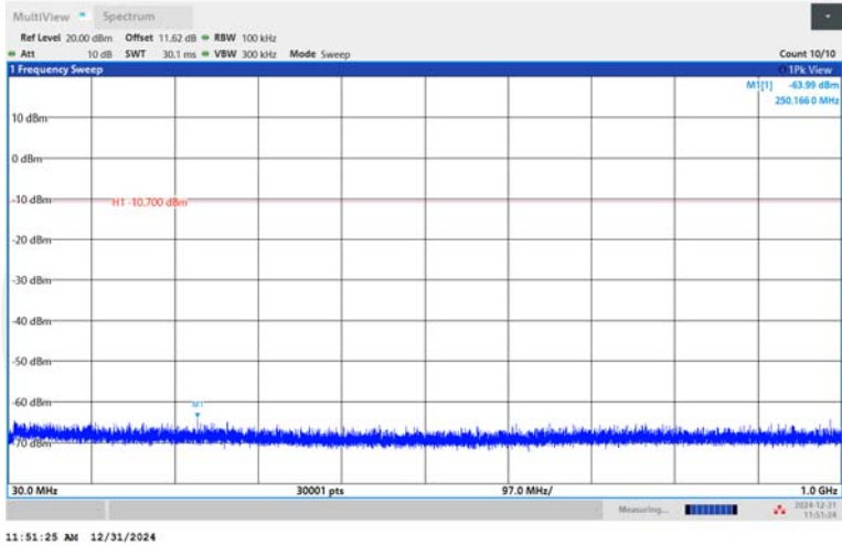
BLE_2M-Ant1-2478-30~1000-PASS
